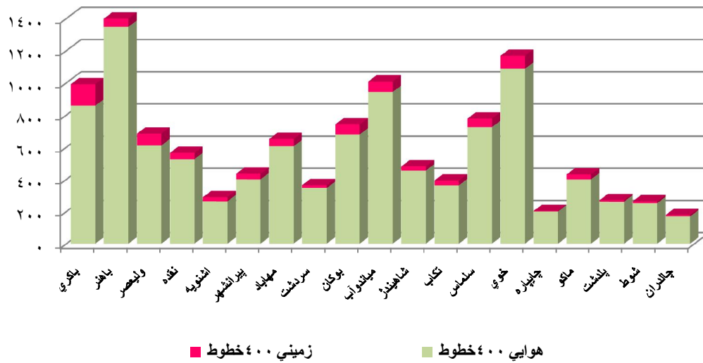
نمودار مقایسه خطوط ۴۰۰ ولت هوایی و زمینی موجود نواحی استان در سال ۱۳۹۲
